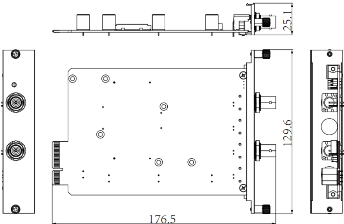
图 3 产品结构尺寸
