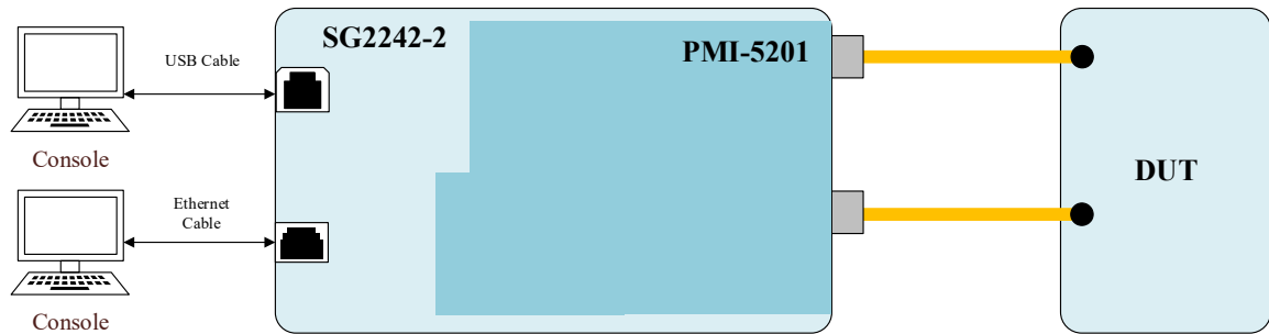
图 1 PMI-5201 典型应用
